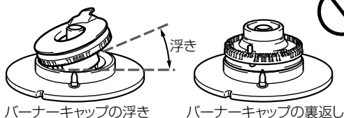
誤ったセットの例
