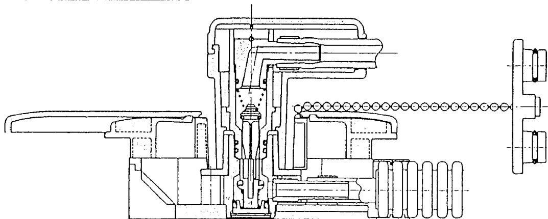
本体・プラグセット図
