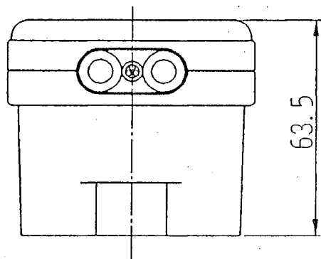
本体・プラグセット図
