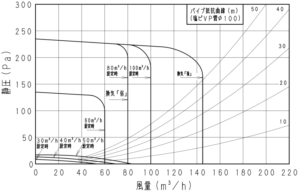
24時間換気「冬期」の風量特性
