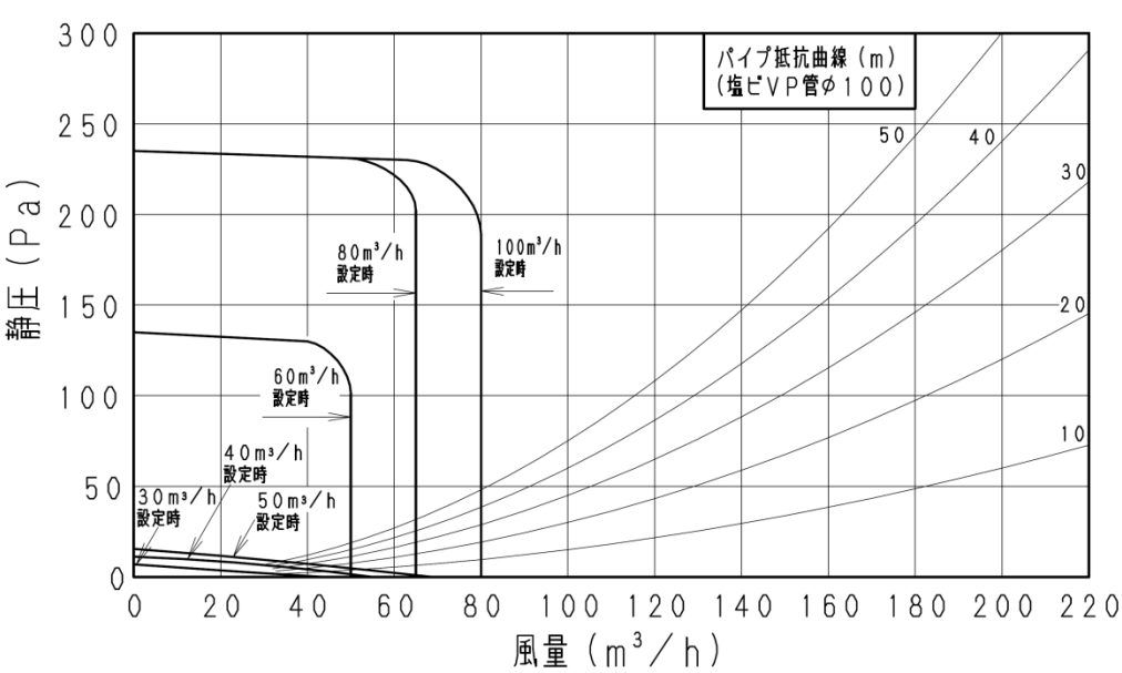
24時間換気「冬期」の風量特性
