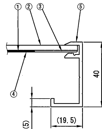
B-B' 断面 (S=1:1)
