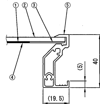
B-B' 断面 (S=1:1)
