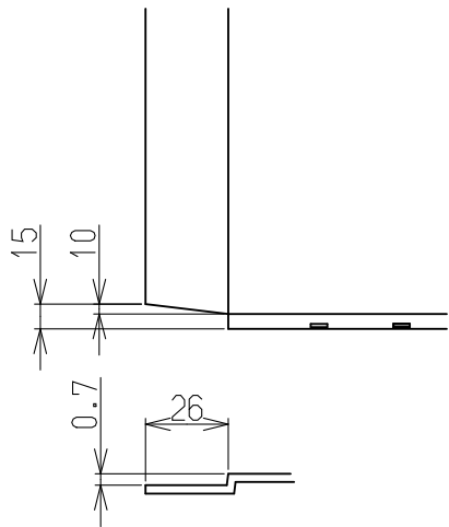
詳細図 B
