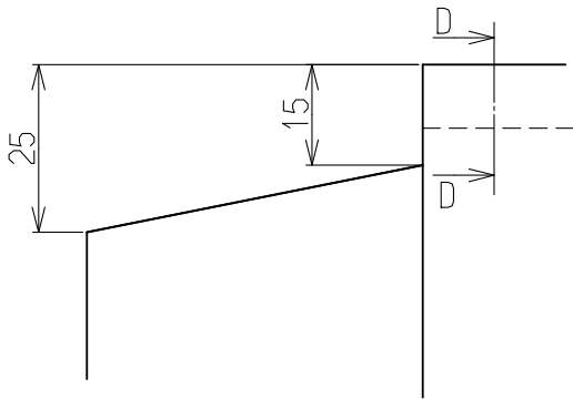
詳細図 A
