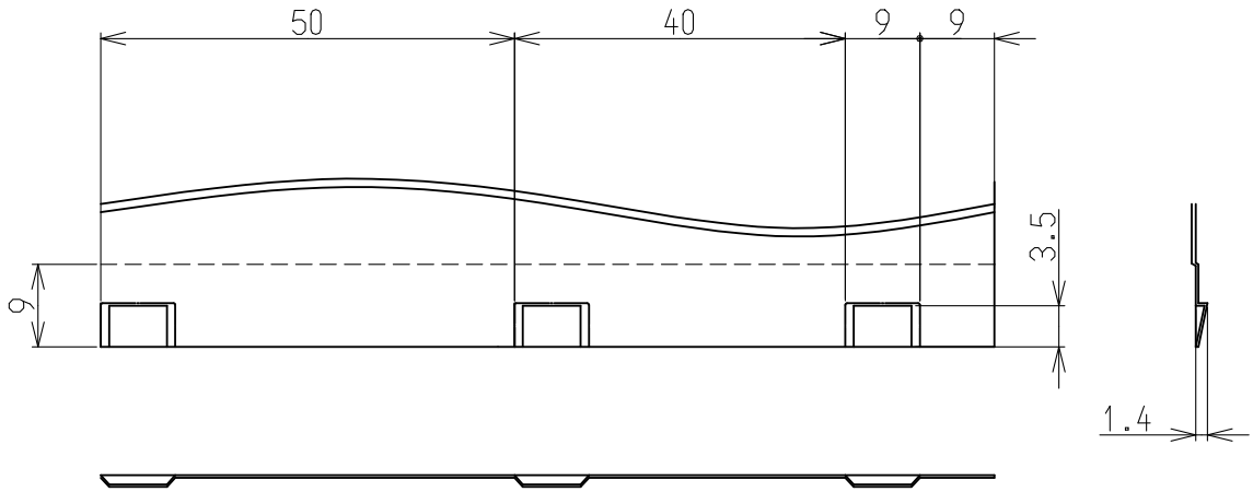
詳細図 C
