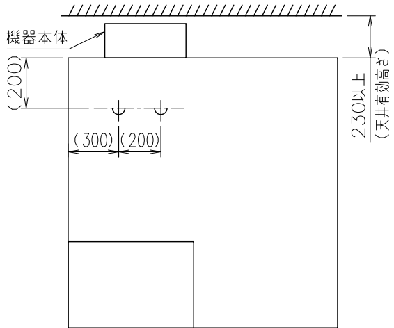
物干しバー収納フック取付 天井有効高さ関係寸法図
