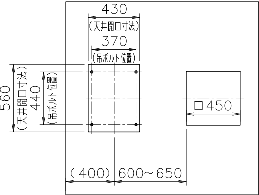
天井開口、吊ボルト、関係寸法図
