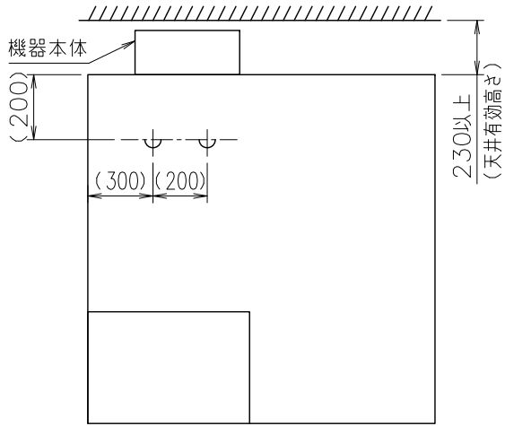
物干しバー収納フック取付 天井有効高さ関係寸法図
