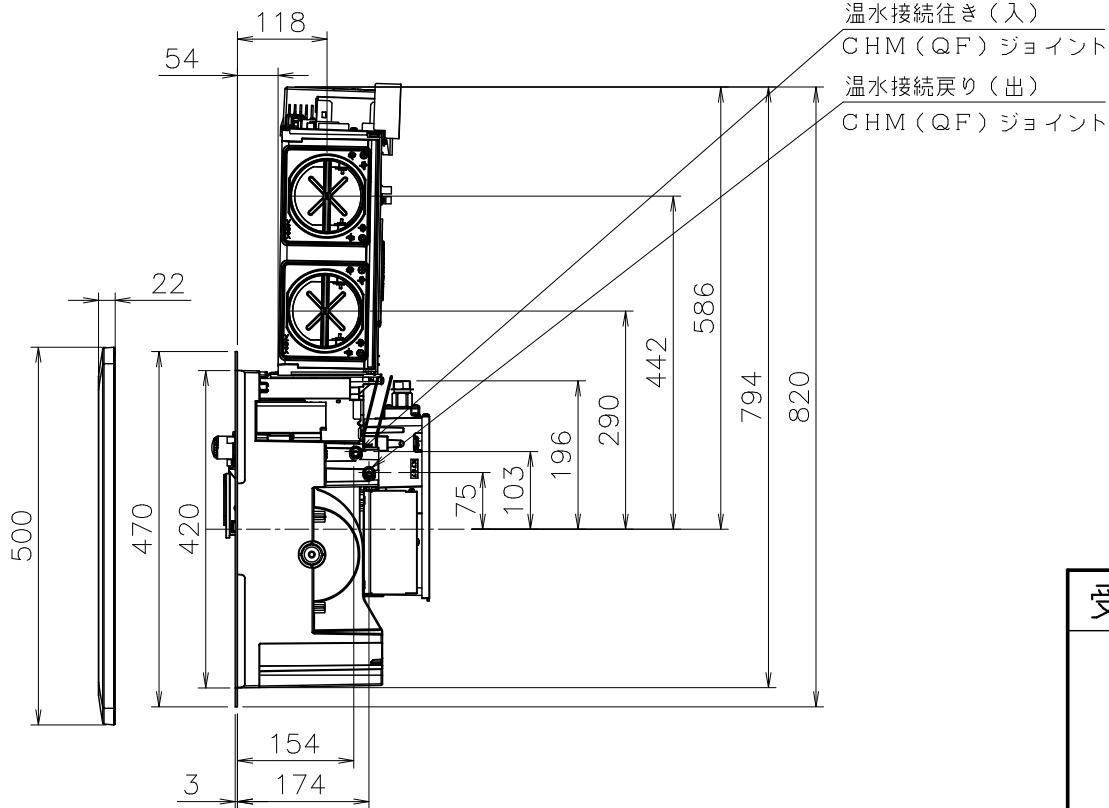
物干しバー収納フック取付 天井有効高さ、配管逃がし関係寸法図
