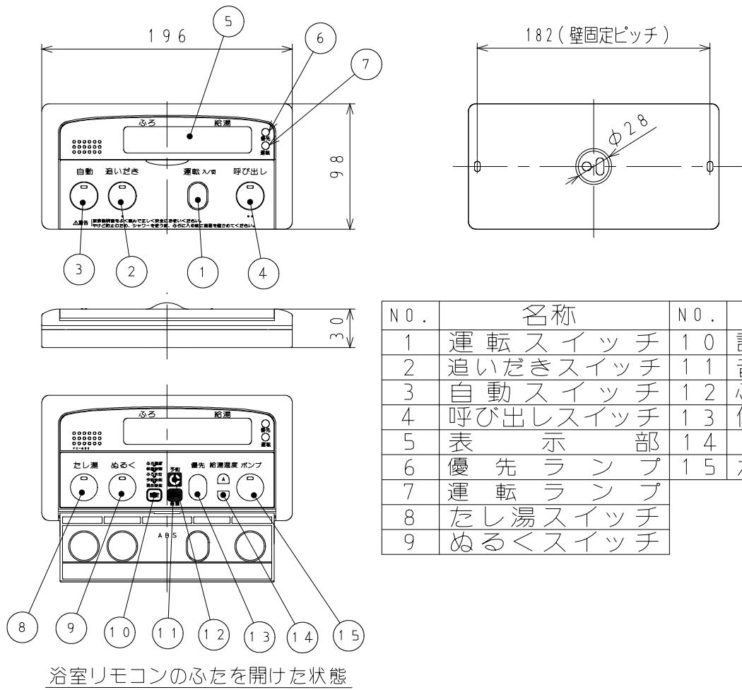
①浴室リモコン寸法図 F C - 6 1 0 ( 単位 : mm )
