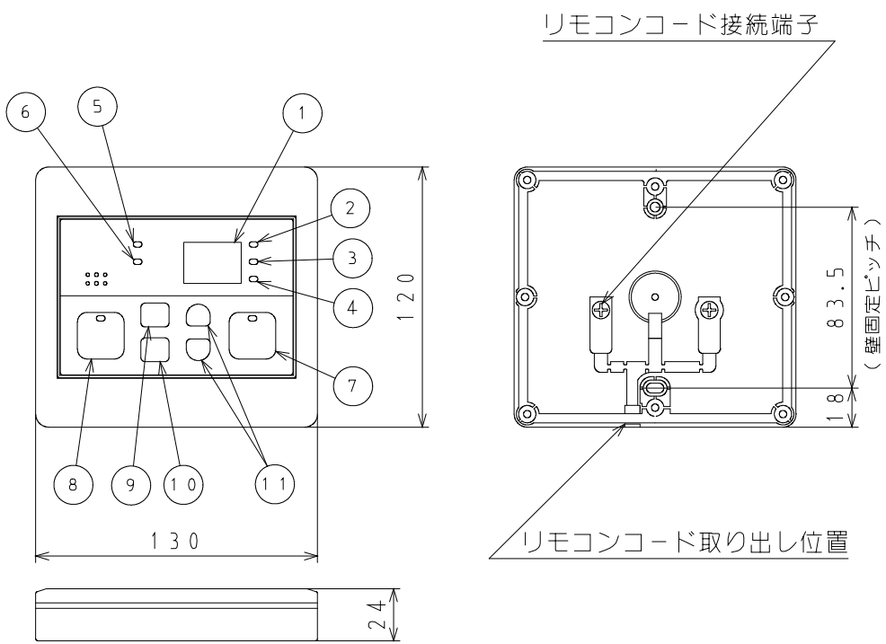
②台所リモコン寸法図 M C - 6 1 0 ( 単位 : mm )
