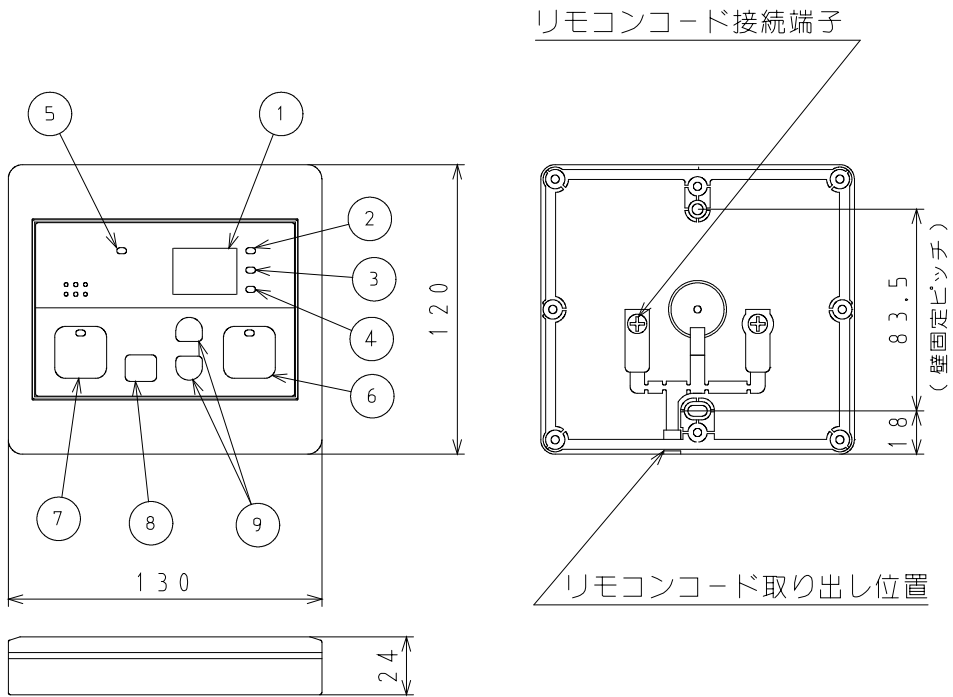
③増設リモコン寸法図 S C - 6 1 0 ( 単位 : mm )
