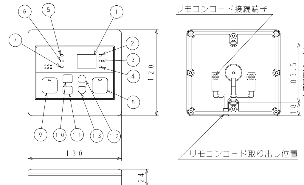
②台所リモコン寸法図 MC-611 (単位: mm)
