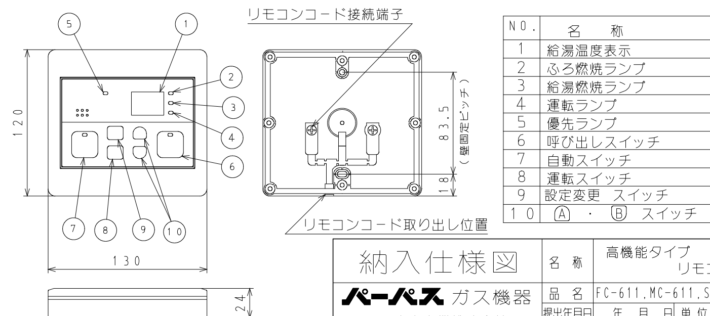
③増設リモコン寸法図 SC-611 (単位: mm)
