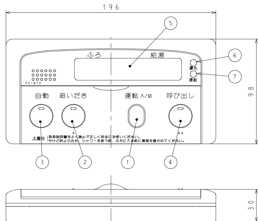
浴室リモコン寸法図 F C - 6 1 3 ( 単位 : mm )
