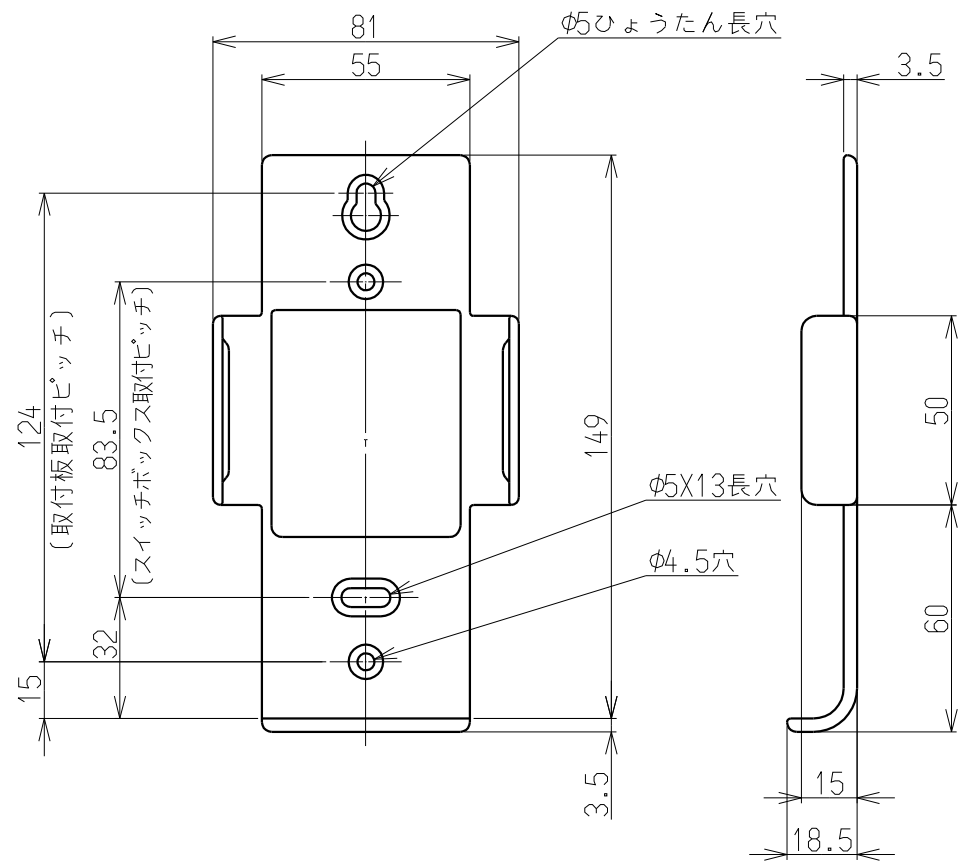
〔取付板〕
