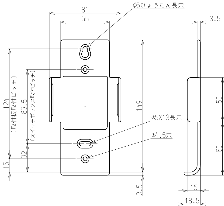
〔取付板〕
