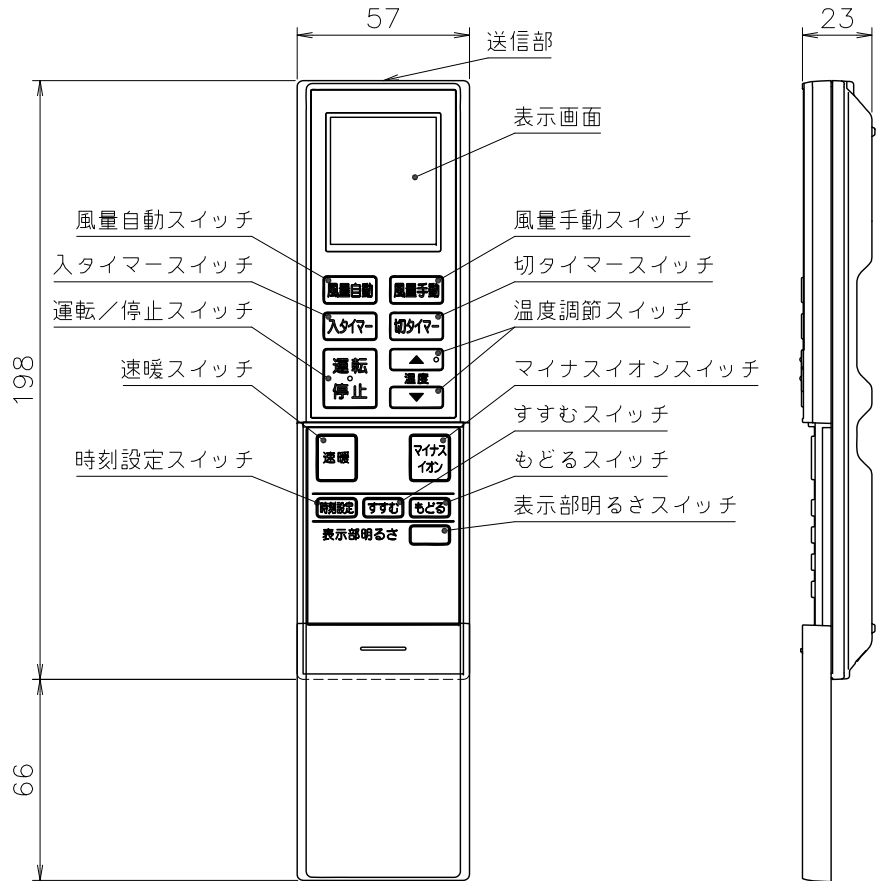
■リモコンRCA-897M(-G)(付属部品)(尺度ー) ふたを開けた状態
