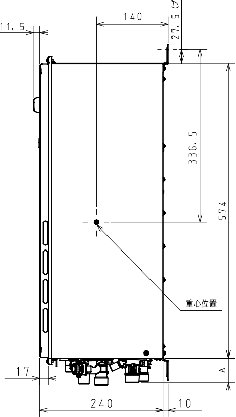
機器底面より各接続口までの寸法
