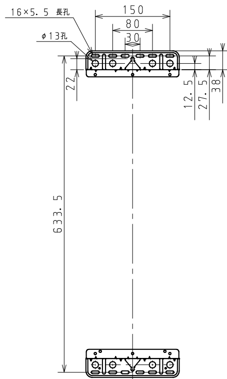
ブラケット
