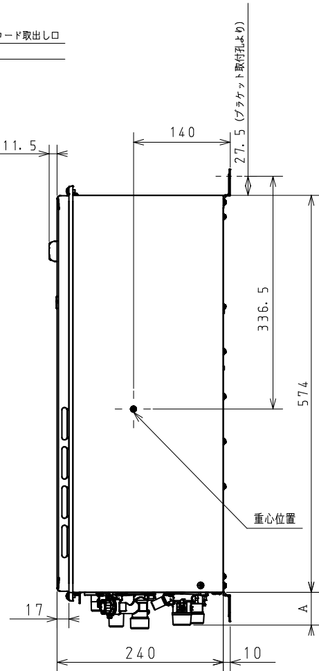
機器底面より各接続口までの寸法
