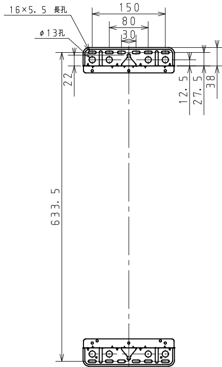
ブラケット
