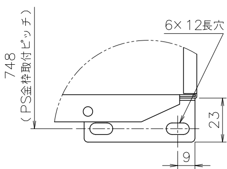
■B部詳細図(尺度1/2)
