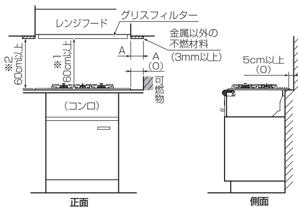
レンジフードおよび不燃材の場合
