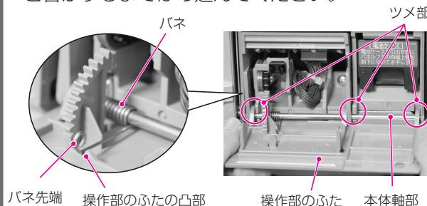
バネ先端 操作部のふたの凸部 操作部のふた 本体軸部
