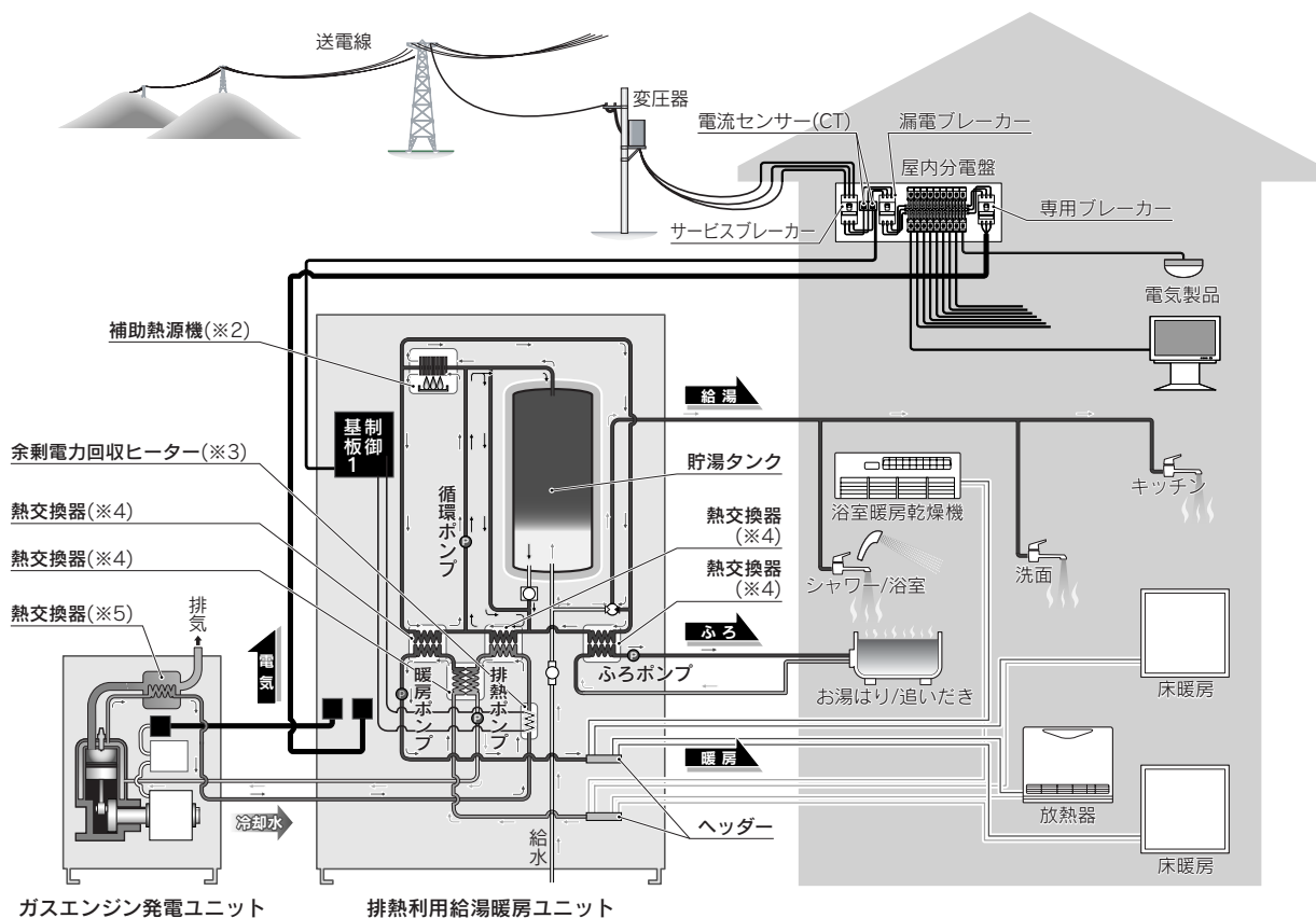
ガス発電・給湯暖房機のしくみ (※1)
