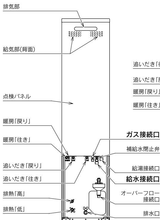
機器上方よりの透視図
