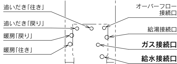
配管位置図
