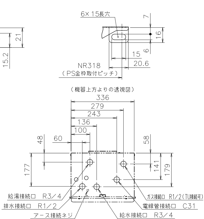
■イ部詳細 (S=1/2)
