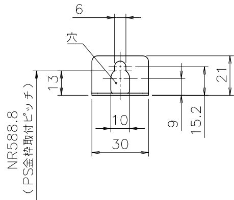
■ア部詳細 (S=1/2)
