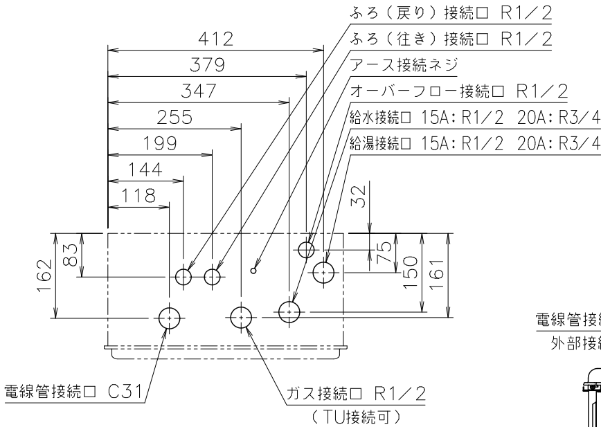
( 機器上方よりの透视图 )
