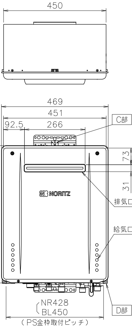
■アルコーブ取付図
