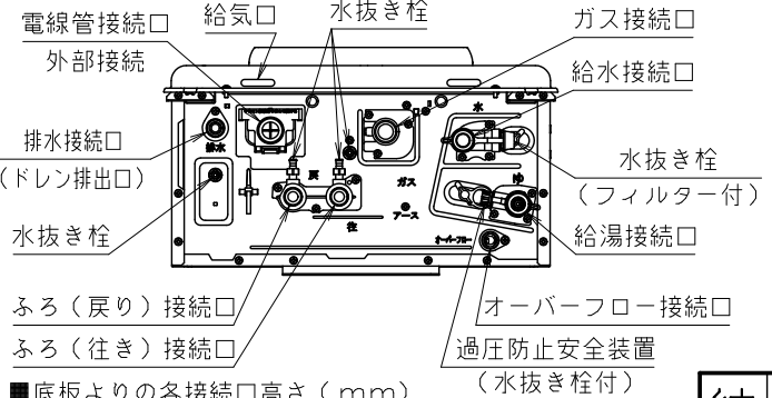
■底板よりの各接続口高さ (mm)
