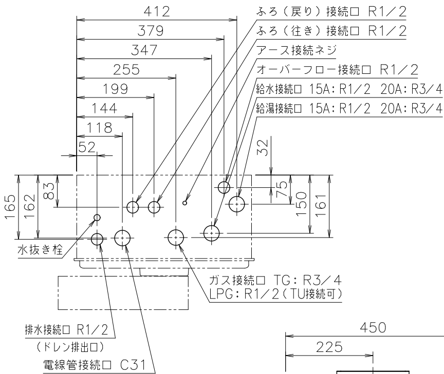
（機器上方よりの透視図）
