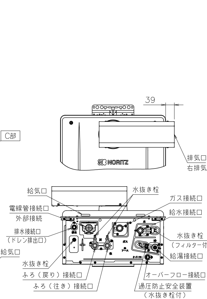
■底板よりの各接続口高さ（mm）
