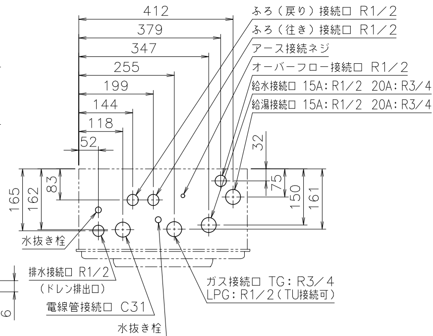
（機器上方よりの透視図）
