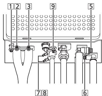
壁掛形 (例: GT-CP2452AWX-PS-2)
