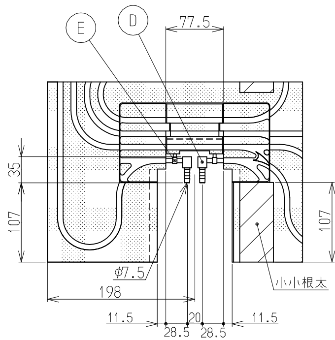
ヘッダー部詳細図
