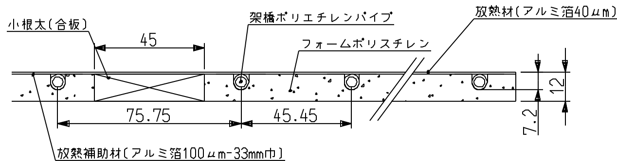
断面詳細図 1 / 2
