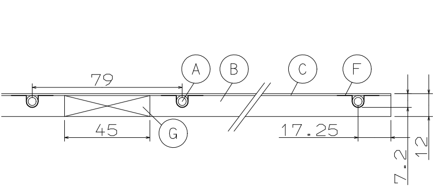
A-A' 詳細図
