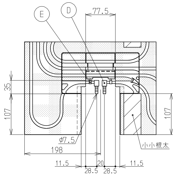
ヘッダ一部詳細図
