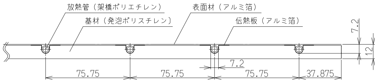
(A-A'断面図)
