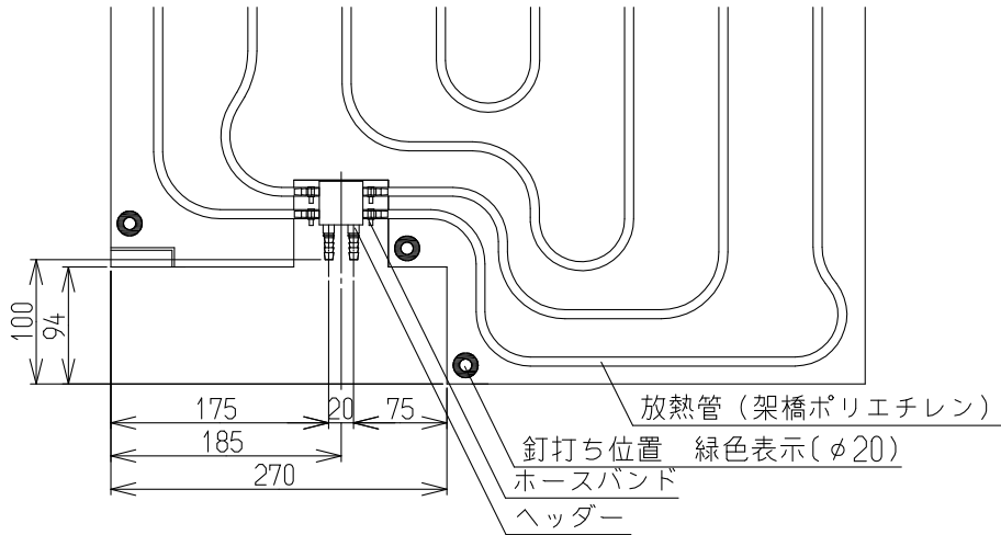
ヘッダー部拡大図
