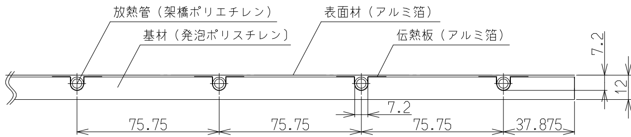
(A-A'断面図)
