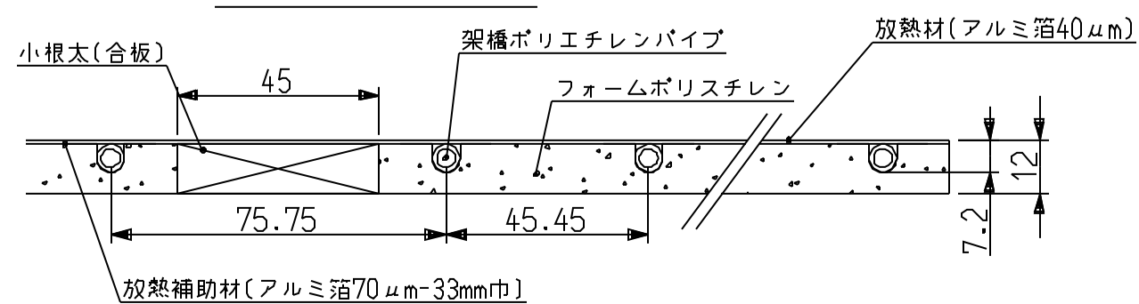
断面詳細図 1 / 2
