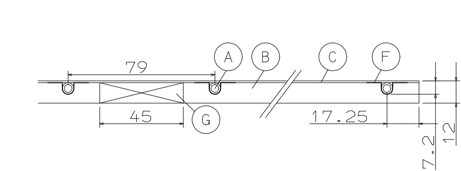
A-A' 詳細図
