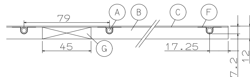
A-A' 詳細図
