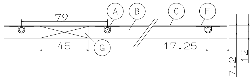
A-A' 詳細図
