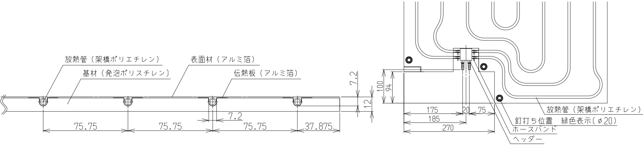
(A-A'断面図)
