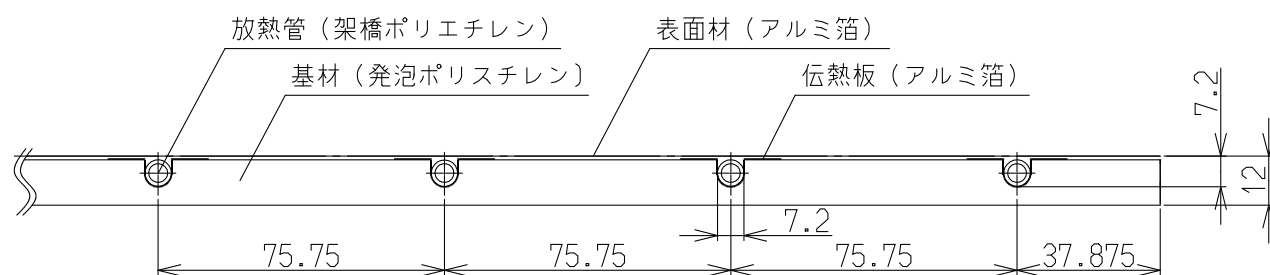
(A-A' 断面图)
