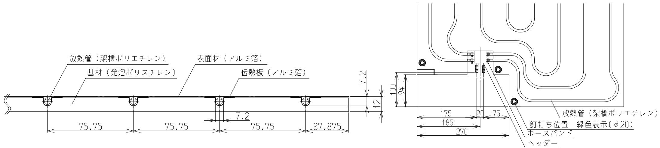
(A-A'断面図)
