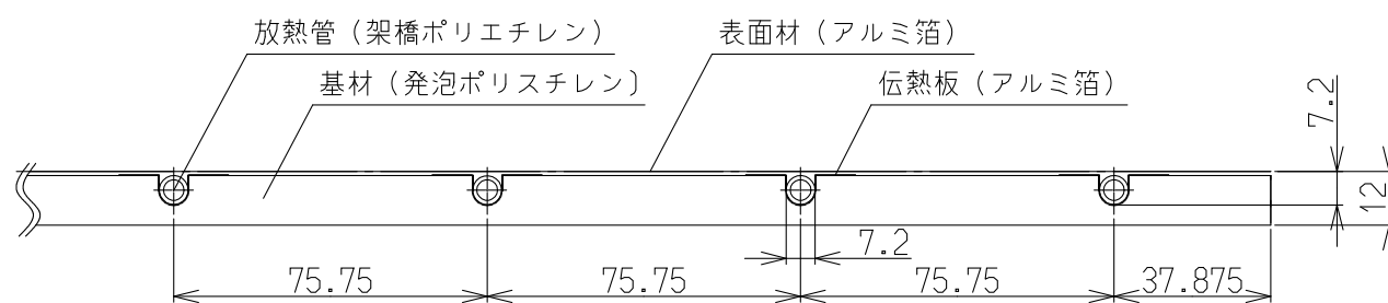
(A-A'断面図)
