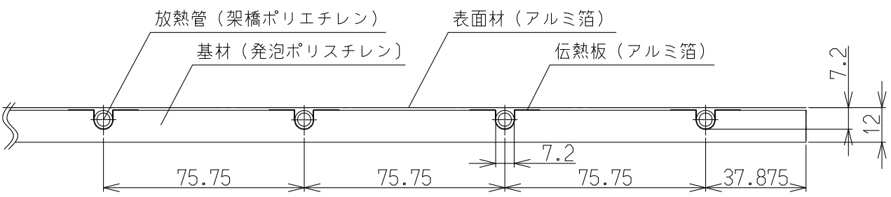
(A-A'断面図)
