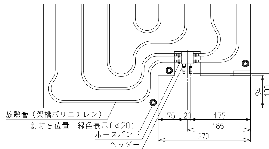
ヘッダ一部拡大図
