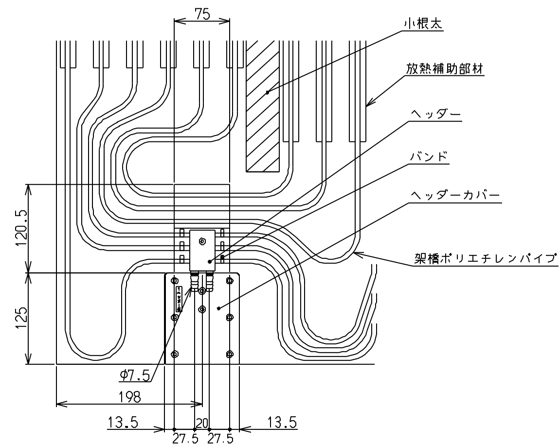
ヘッダー部詳細図
