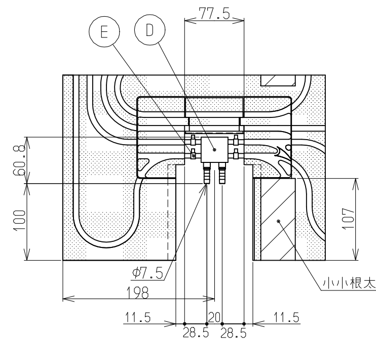
ヘッダー部詳細図
