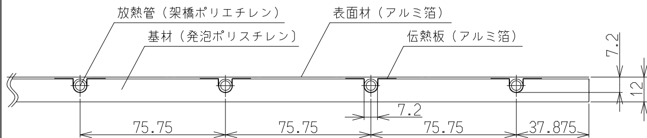
（A－A'断面図）
