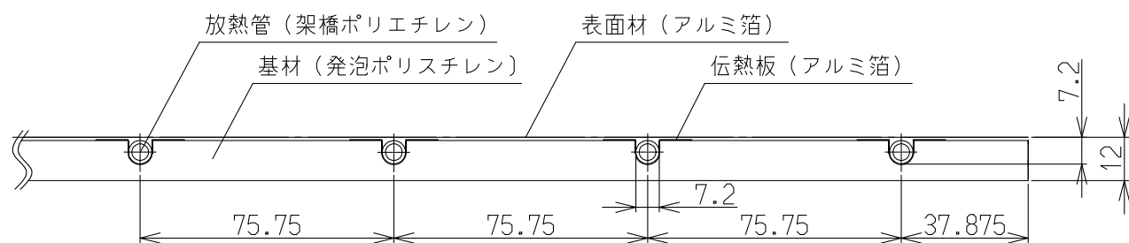
(A-A'断面図)
