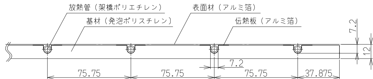
(A-A'断面図)
