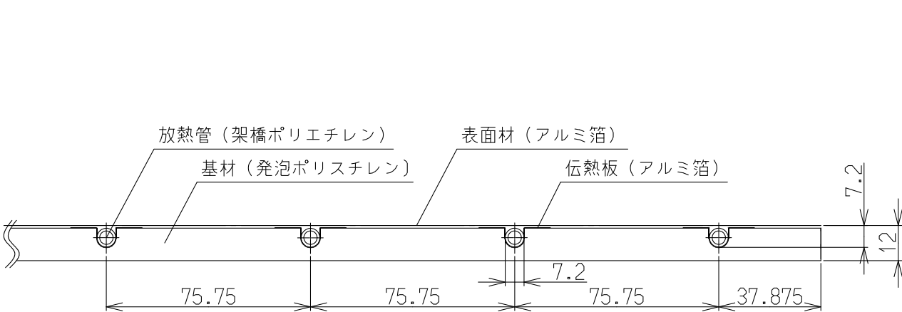
(A-A'断面図)
